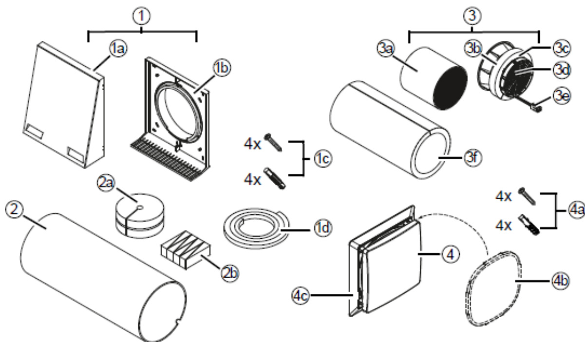
Obrázek 6: komponenty větracího přístroje iV-Office ve standardní variantě.
