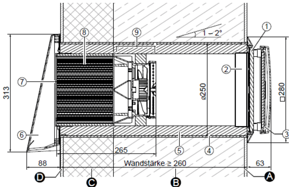
Obrázek 3: průřez větracím přístrojem iV-Office.
