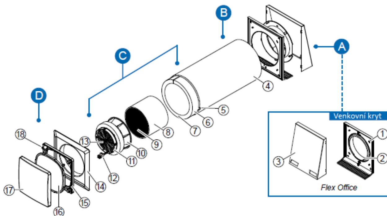
Obrázek 1: konstrukce větracího přístroje iV-Office.
