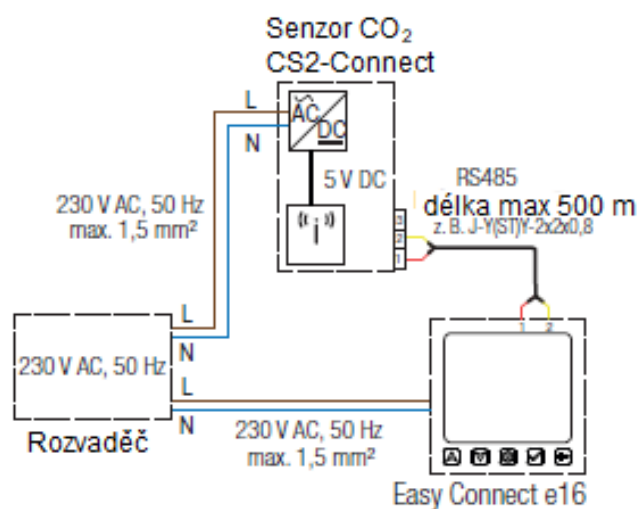
B: Kabelové připojení větracích přístrojů
