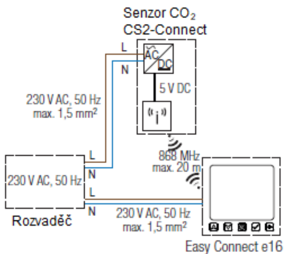
A: Bezdrátové připojení větracích přístrojů
