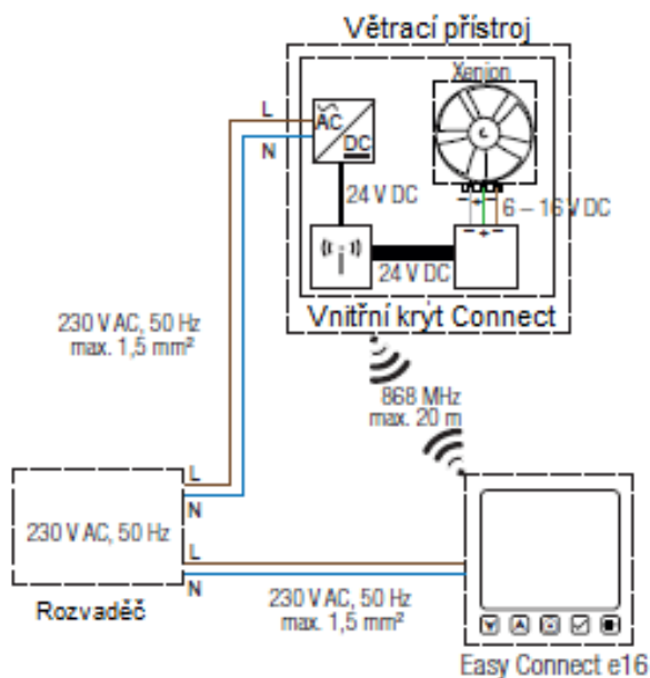
A: Bezdrátové připojení větracích přístrojů
