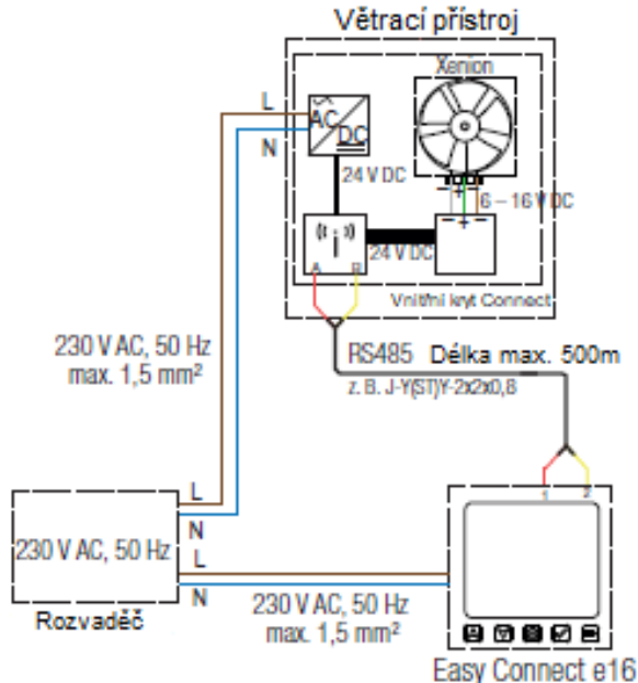
B: Kabelové připojení větracích přístrojů
